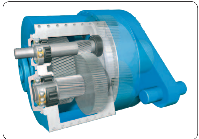
Windturbinengetriebe
