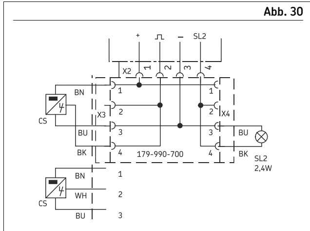
Steckerbelegung
