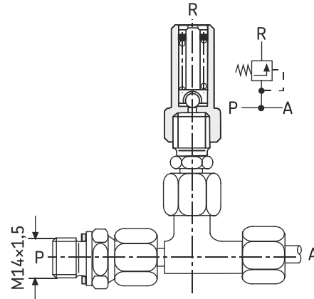
Druckbegrenzungsventil mit T-Stück
