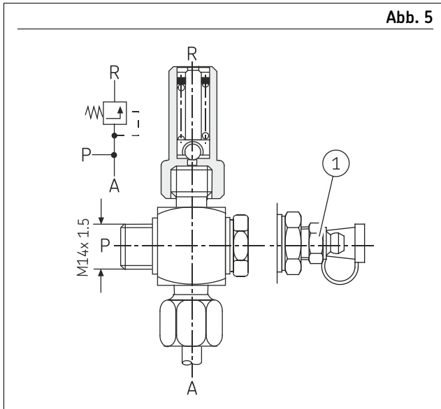
Druckbegrenzungsventil
