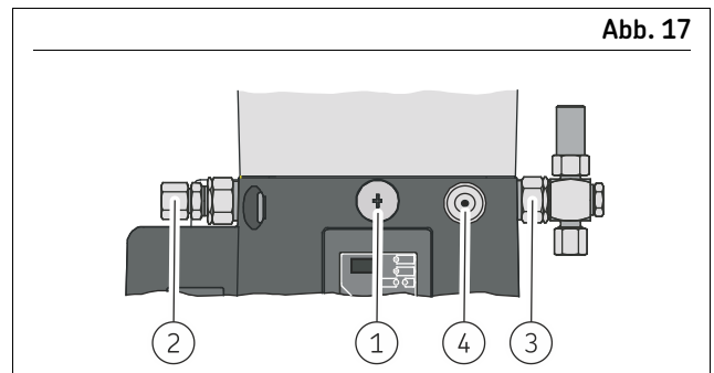
Abbildung 17: Anschluss Pumpenelemente
