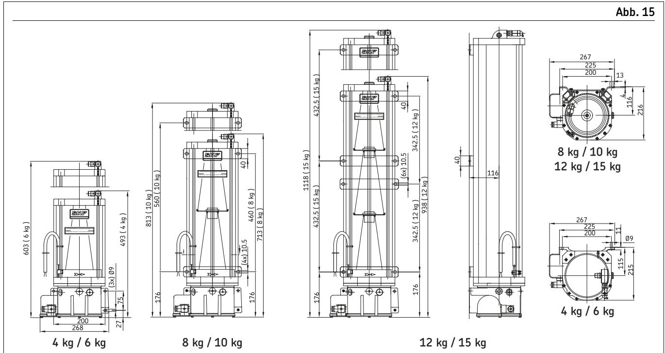
Abmessungen KFG in mm
