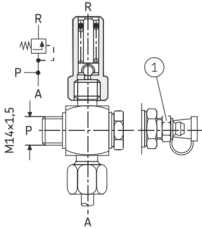
Druckbegrenzungsventil mit Notschmiernippel
