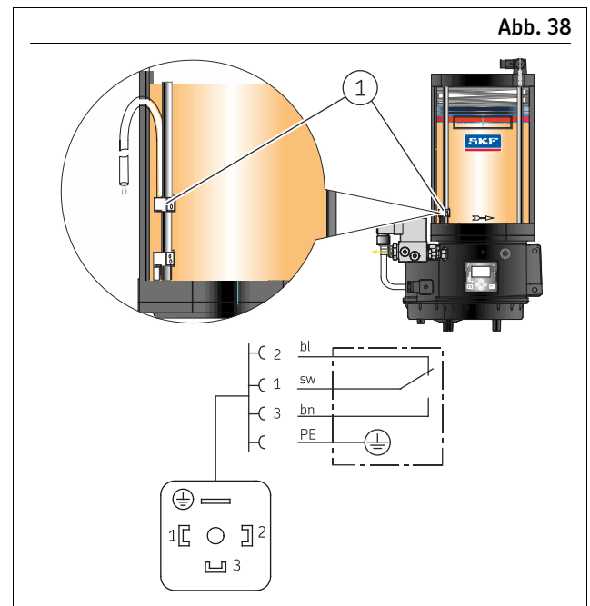
Füllstandsschalter
