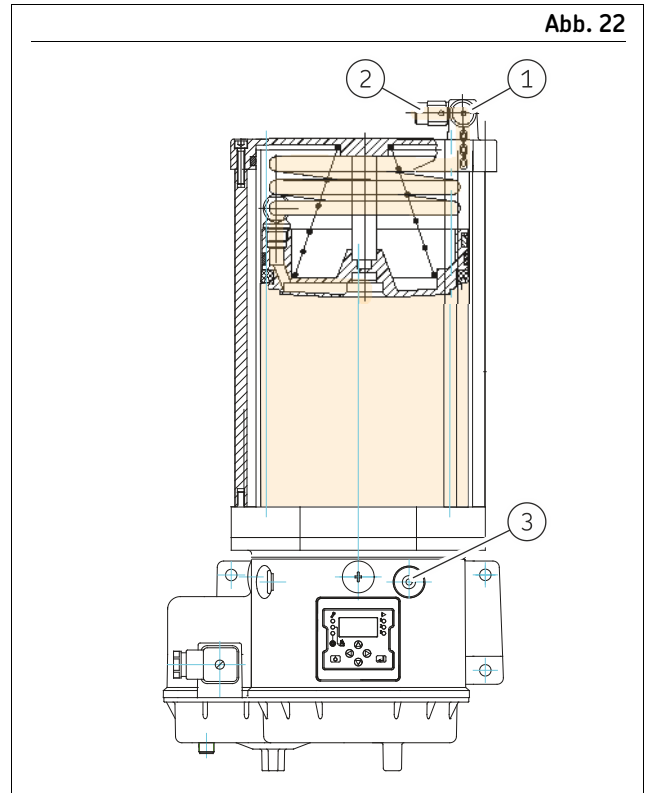
Abbildung 22: Befüllanschluss am Behälterdeckel
