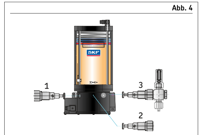
Anordnung der Pumpenelemente
