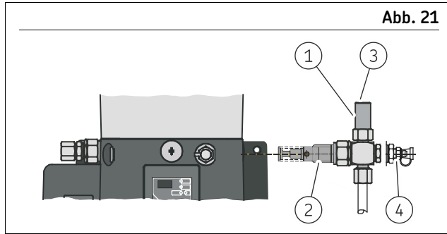
Abbildung 21: Anschluss Druckbegrenzungsventil
