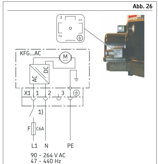
1) Externes Steuergerät Relaiskontakt „Pumpe ein“ Steckerbelegung 230 VAC (90-264 VAC)
