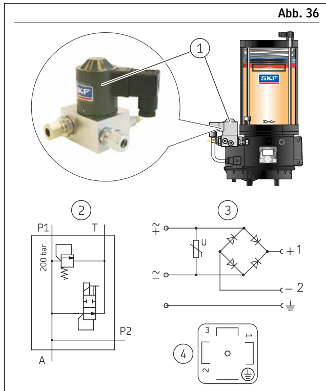
Entlastungsventil/Druckbegrenzungsventil
