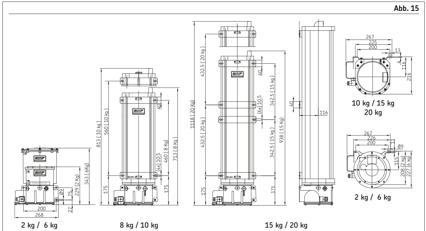
Abmessungen KFG in mm
