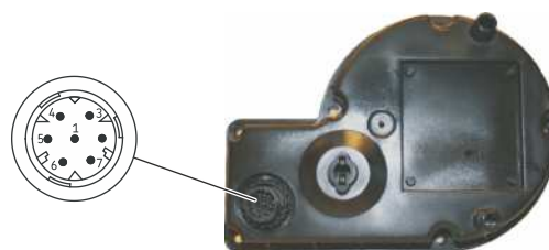
Steckdosenverbindung nach ISO 15170-1
