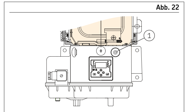
Befüllen über Befüllanschluss
