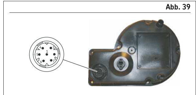
Steckerbelegung Füllstandsüberwachung
