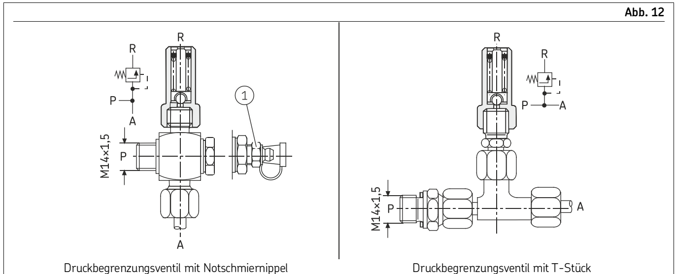
Druckbegrenzungsventil mit Notschmiernippel
