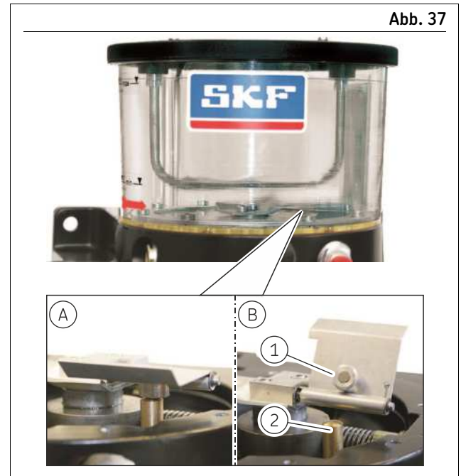
Füllstandsschalter
