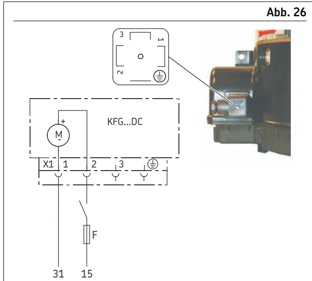
Steckerbelegung 12/24 VDC
