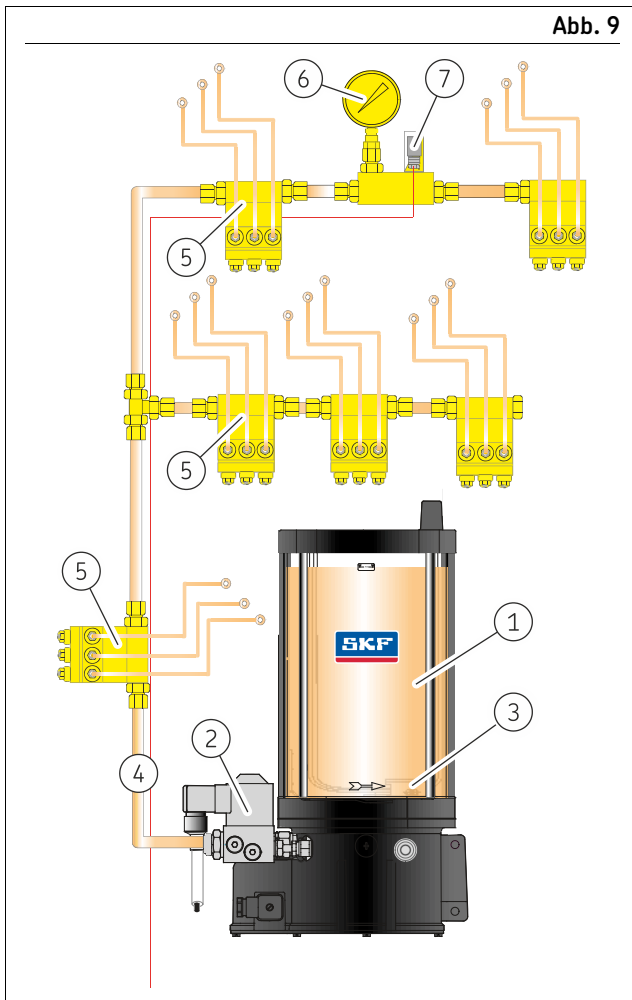
Einleitungsanlage mit KFG-Pumpenaggregat
