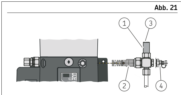
Anschluss Druckbegrenzungsventil
