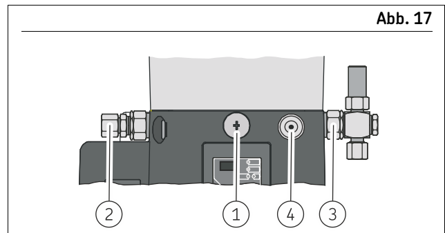
Anschluss Pumpenelemente
