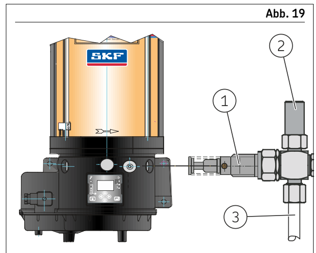
Montage, federrückgeführtes Pumpenelement
