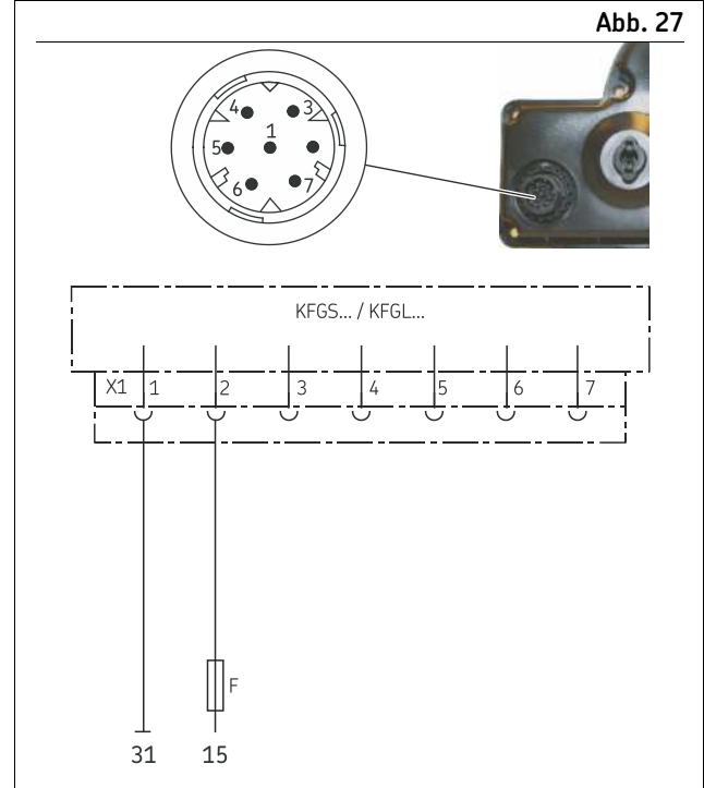
Steckerbelegung 12/24 VDC
