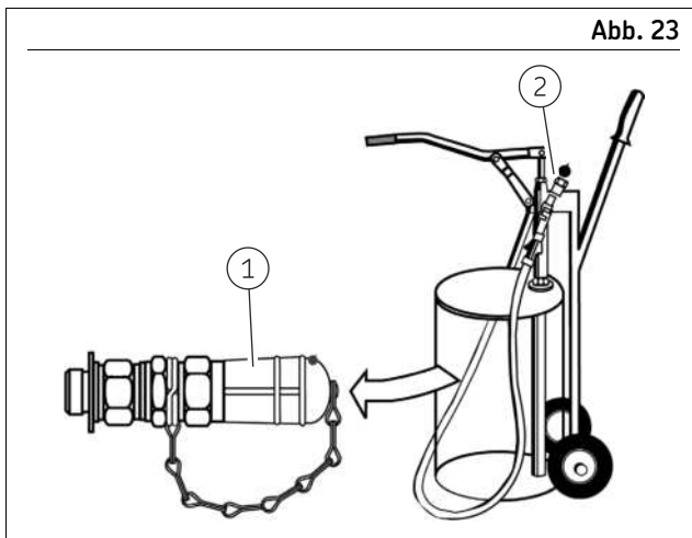
Befüllkupplung (Option)
