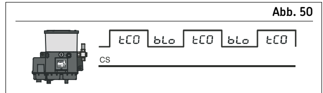
Fehlendes Signal vom Kolbendetektor
