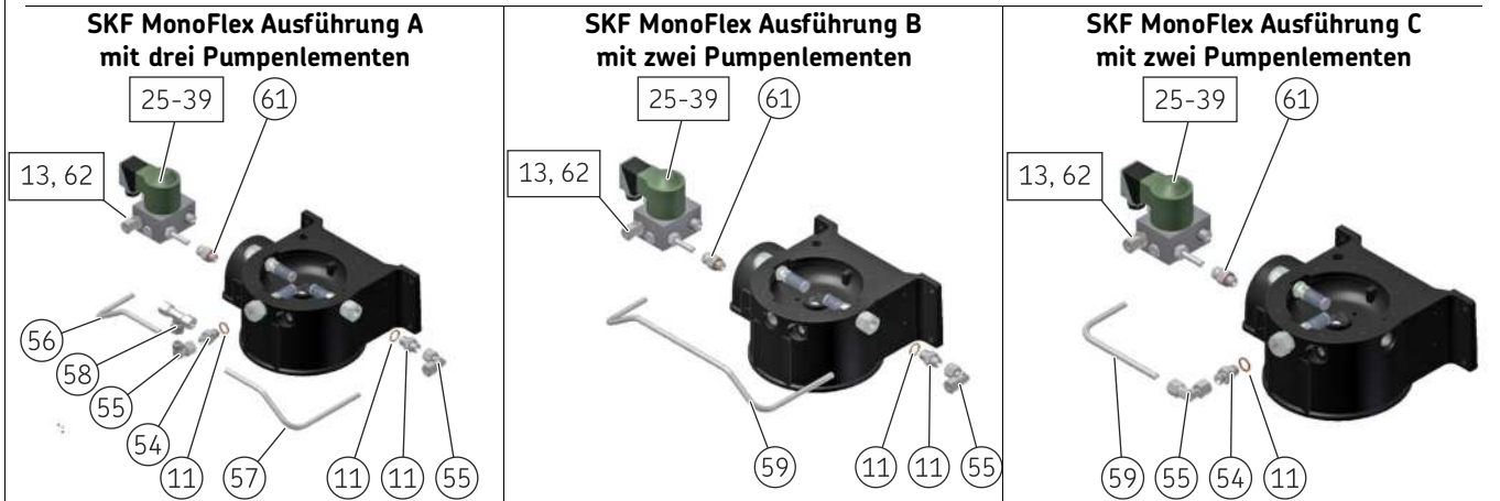
Explosions- und Ersatzteilzeichnung
