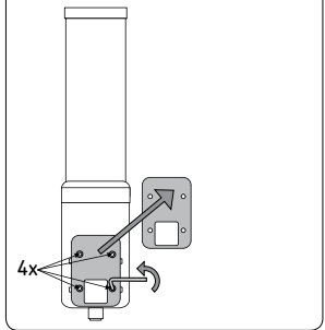
Az elemtartó rekesz fedelének visszaszerelése
