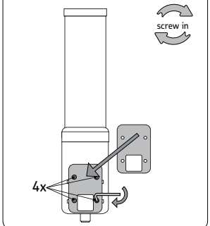
Az elemtartó rekesz fedelének visszaszerelése
