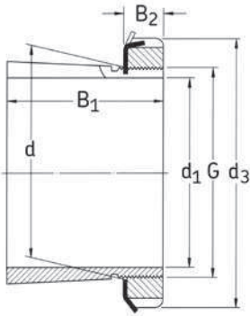
Type HA, HE, HS
