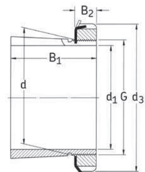
Type HA, HE, HS
