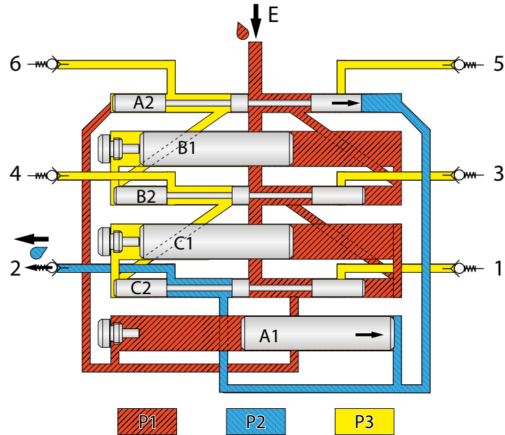
Abb.14 Schmierstoffverlauf am Beispiel eines SSVD-6 Verteilers Phase 5 und 6
