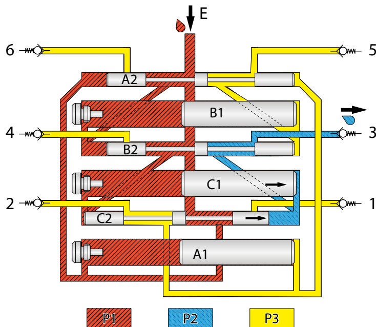
Abb.16 Schmierstoffverlauf am Beispiel eines SSVD-6 Verteilers Phase 9 und 10
