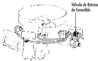
FIGURA 12: VÁLVULA DE RETRASO DE ENCENDIDO TÍPICA
