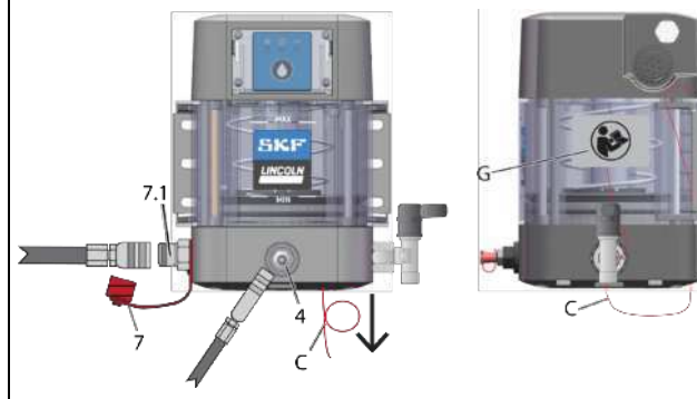
Erstmaliges Befüllen einer leer gelieferten Pumpe
