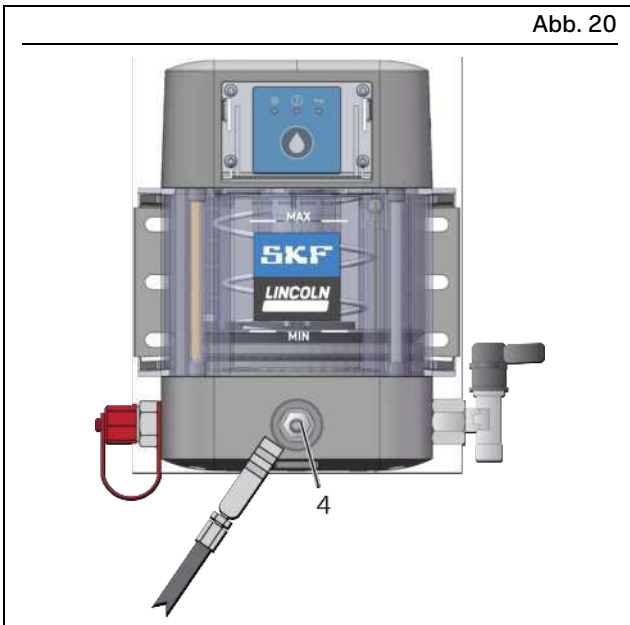
Regelmäßiges Befüllen mit Befüllnippel
