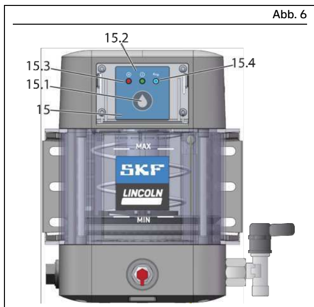
Pumpengehäuse Oberteil
