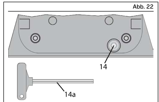
Entlüftungsrohr reinigen
