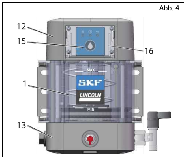
CLP Pumpe Vorderansicht
