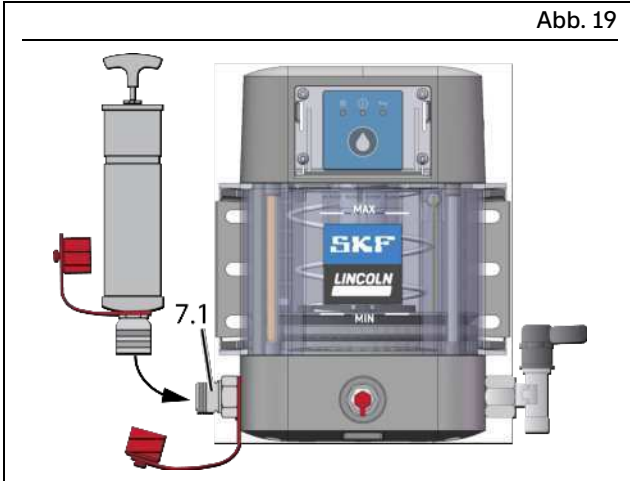
Regelmäßiges Befüllen mit Kartusche
