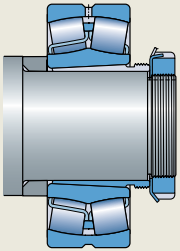
通过推卸套安装在阶梯轴上的圆锥孔轴承
