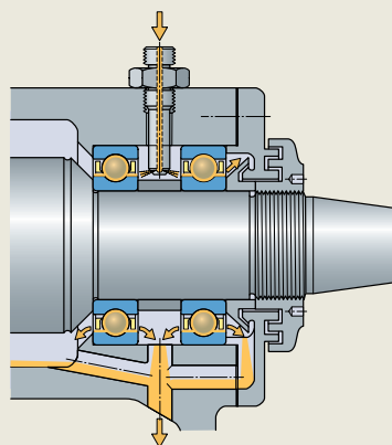
喷油润滑
