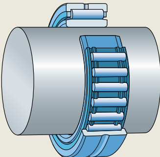
带机削套圈的滚针轴承
