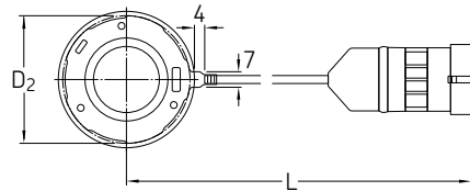
BMD ... 108A (Superseal™ 接头)
