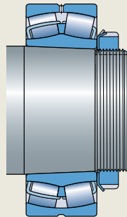
图 3 安装在圆锥形轴颈上的带圆锥孔轴承
