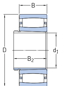
AH 推卸套 上的轴承
