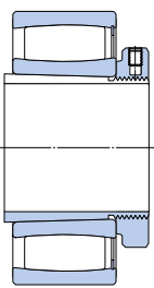
H..E 紧定套上的轴承
