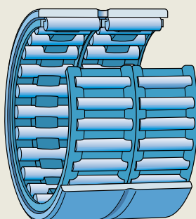
不带挡边的双列滚针轴承
