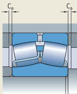
轴承两侧的自由空间
