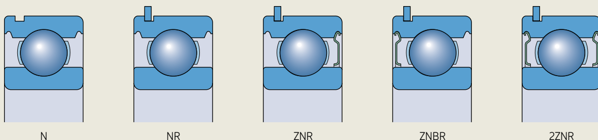
带止动槽不同型式的轴承
