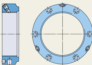
KMTA 锁紧螺母在圆周上和一侧端面有孔
