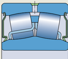
装在外圈凹槽中的密封
