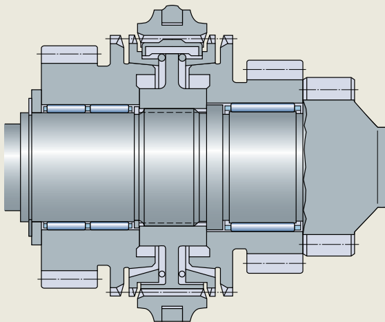
分体式保持架的滚针和保持架组件
