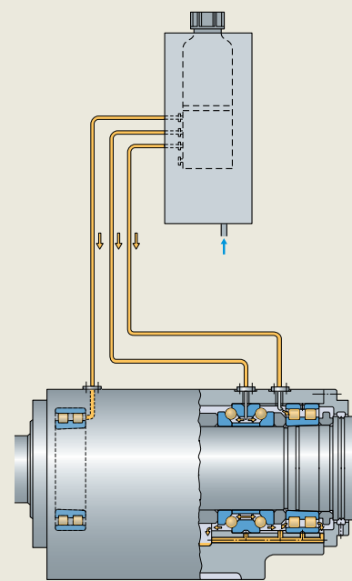
油气润滑
