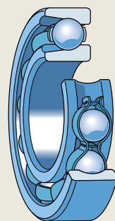
带装球缺口的轴承
