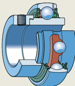
YEL 2 系列轴承
