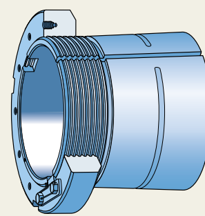
带螺母和防松片的紧定套
