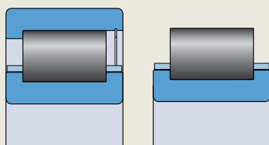
NCF ..ECJB
