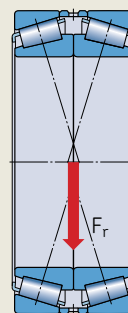
面对面配置的配对轴承的径向载荷
