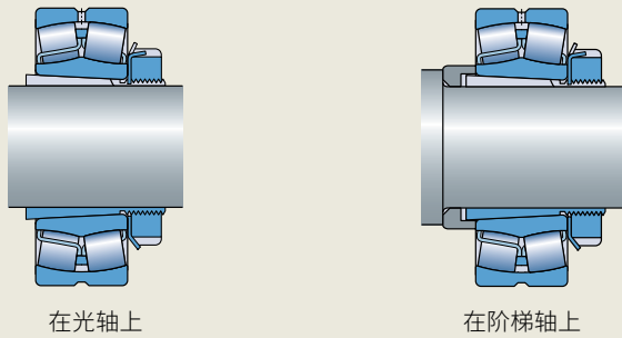
通过紧定套安装圆锥孔轴承
