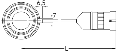
BMB ... 108A (Superseal™ 接头) BMO ... 108A (Superseal™ 接头)
