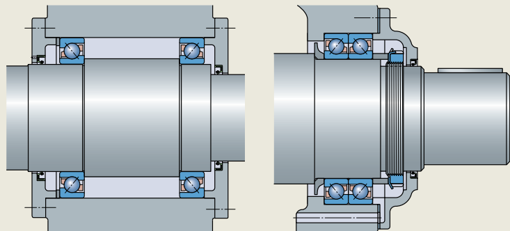
面对面配置的单个轴承
