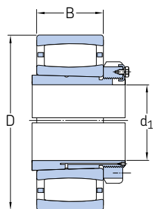
OH..H 紧定套 上的轴承
