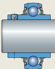
采用紧定螺钉锁定的轴承
