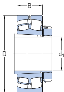
H.. 紧定套上的 轴承
