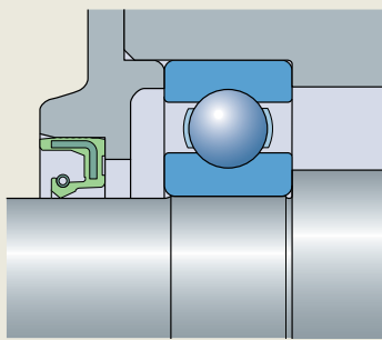
图 15 安装径向轴密封，防止污染物进入
