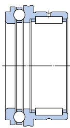
NKX (F w ≥ 12 mm)
