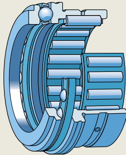
与带保持架的推力轴承组合，NKX
