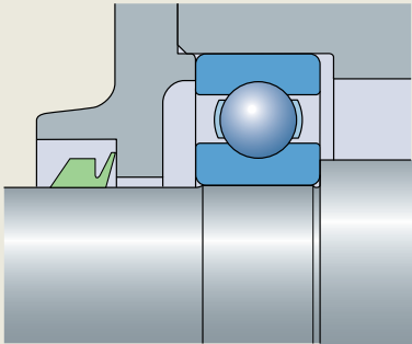
V形密封
