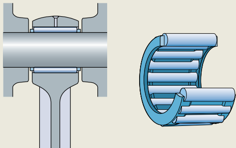
安装在活塞销（十字头销）上的特殊滚针和保持架组件
