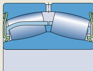
用卡环固定的密封
