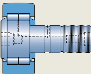
NUKR .. A 型
