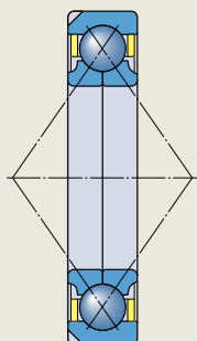
带定位槽的四点接触轴承
