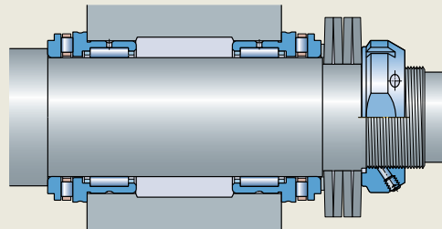
背对背安装的带碟形弹簧的 NKXR 系列轴承
