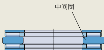
双向轴承, 轴承座引导
