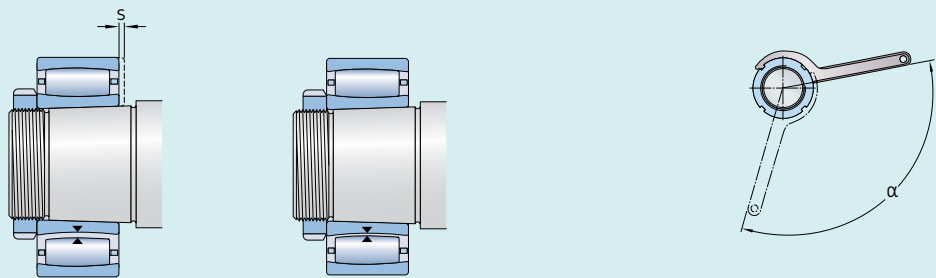
带圆锥孔的 CARB 轴承的推进参数
