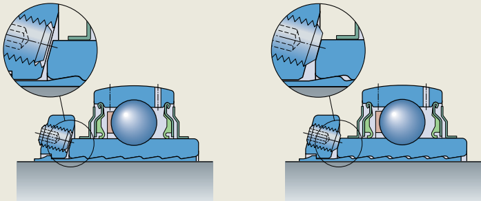
SKF ConCentra 锁定技术
