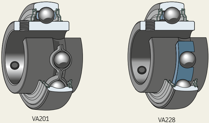
高温外球面轴承的几种变型
