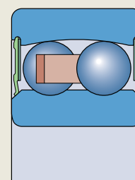
两侧带接触式密封
