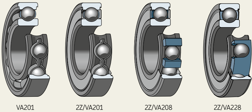
高温深沟球轴承的几种变型
