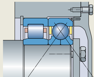
图 2 圆柱滚子轴承与四点接触球轴承的组合
