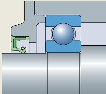
图 14 安装径向轴密封，防止润滑油泄漏
