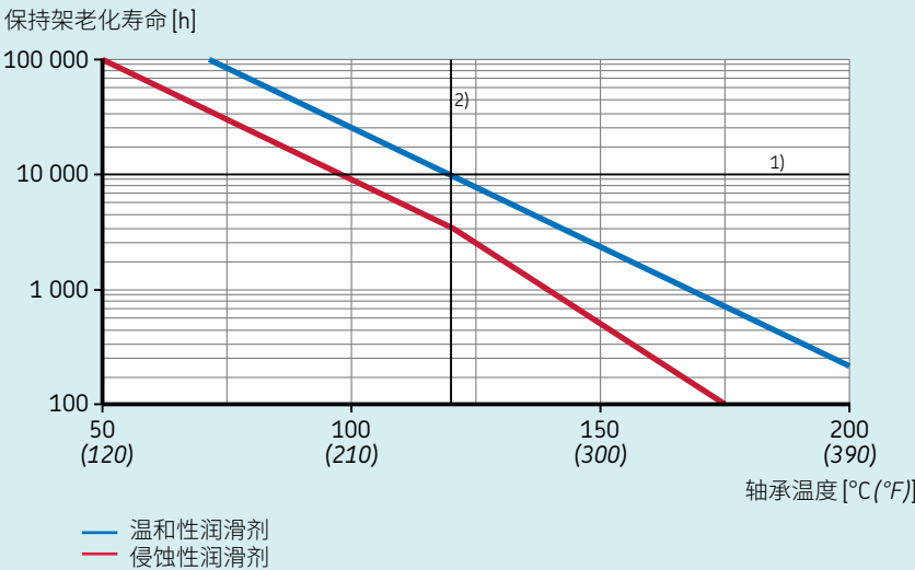
玻璃纤维增强尼龙 PA66 的老化寿命
