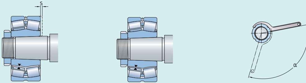
带圆锥孔的球面滚子轴承的推进数据
