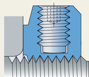
使用紧定螺钉锁定 — KMFE
