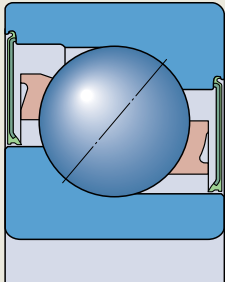
闭式轴承 — 非接触式密封
