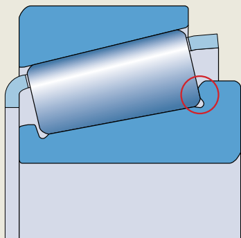
滚子端面与挡边接触处
