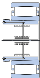
AOH 推卸套 上的轴承
