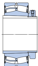
H..E 紧定套上 的密封轴承
