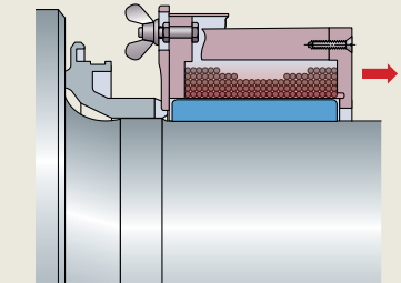
特殊固定感应加热器
