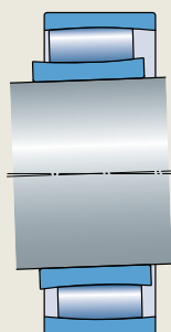
CARB 圆环滚子 轴承
