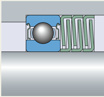
SKF 密封组圈
