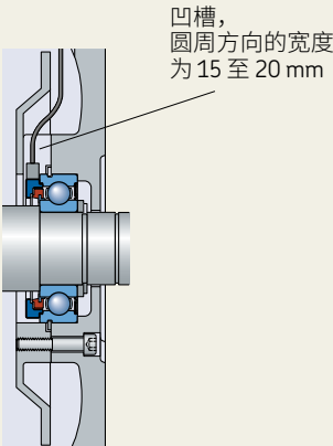
轴承座内径向凹槽
