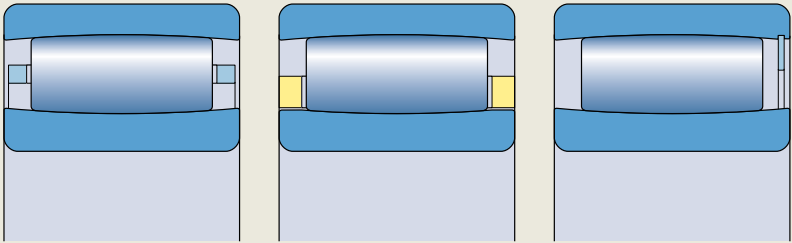
滚动体引导保持架的轴承
