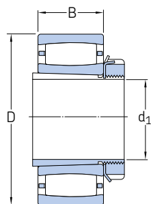
H.. 紧定套上的轴承
