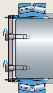
借助注油法安装在退卸套上
