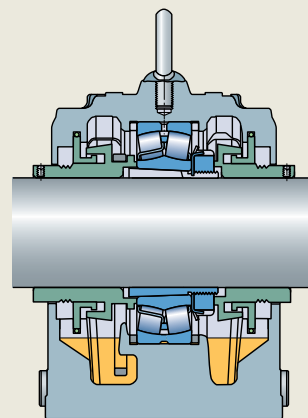
SONL 轴承座内的甩油环
