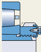
E (带 HME 螺母)
