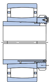
OH..HE 紧定套 上的轴承
