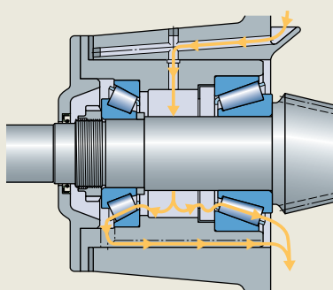
通过排油管和油道实现润滑油自循环
