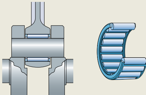
安装在曲柄销（曲轴轴颈）上的特殊滚针和保持架组件
