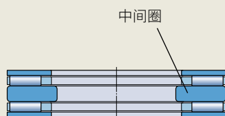
双向轴承, 轴引导
