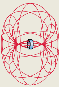
以 CARB 轴承外圈轴线回转所得的圆环滚道面
