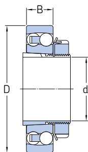
标准紧定套上的 开式轴承
