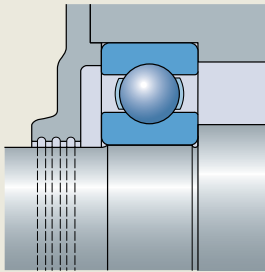
外置带同轴槽间隙式密封
