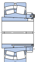
OH ..H 紧定套上的 轴承
