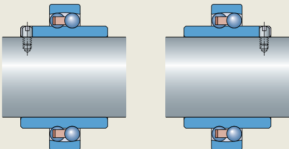
内圈加长轴承的轴向定位
