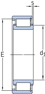
NCF ..ECJB
