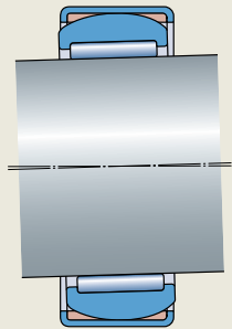
调心滚针轴承
