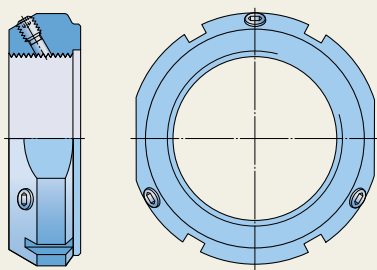
两侧带对称铰平的 KMT 锁紧螺母
