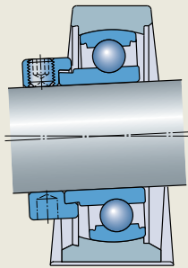
球轴承单元
