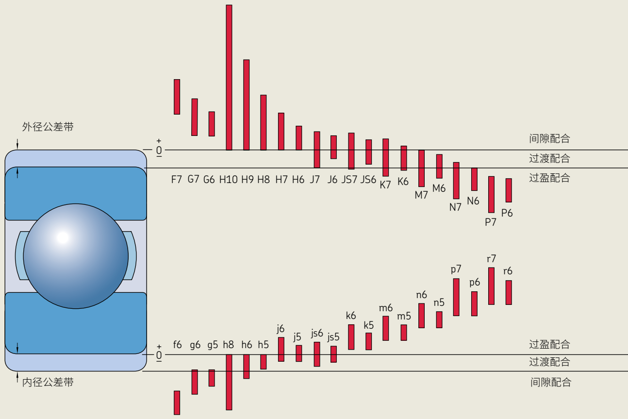
轴和轴承座公差等级的位置和范围
