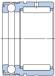
NX (F w ≥ 10 mm)
