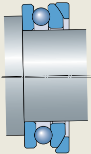
带调心座圈的推力球轴承
