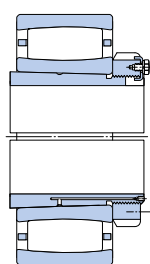
OH..H 紧定套上的轴承
