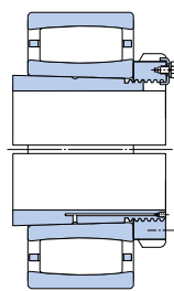
OH..H 紧定套上的轴承
