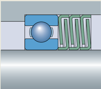
SKF 组合迷宫密封
