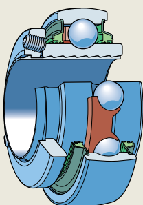
YSPAG 2 系列轴承
