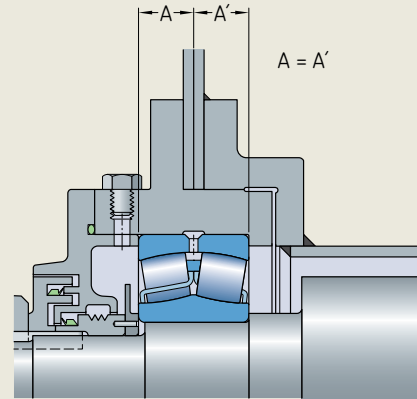
将轴承中心与振动筛机架中心对齐
