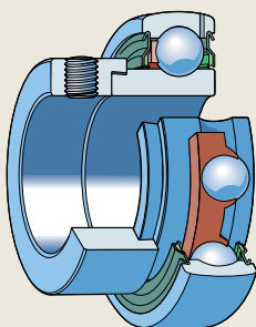
YET 2 系列轴承
