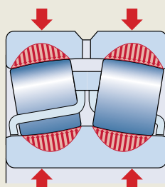
沿滚子长度方向的载荷分布
