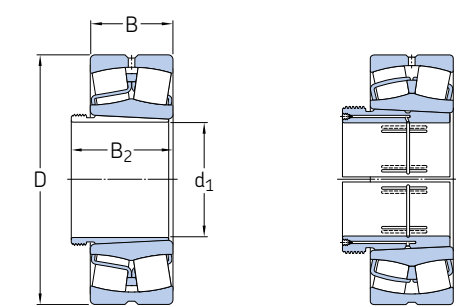
AH 轴套上的轴承
