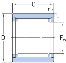
NK (F w ≤ 10 mm)
