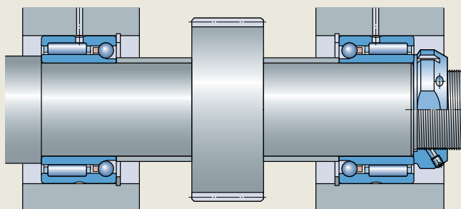
背对背安装的NKIA系列轴承
