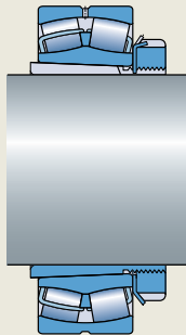
图 2 用紧定套安装在光轴上的带圆锥孔轴承
