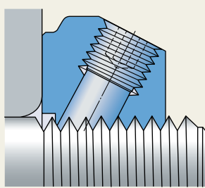
使用防松销锁定
