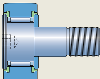
KR .. PPSKA 型
