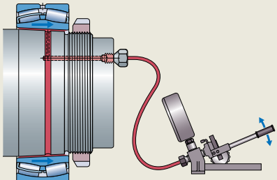
借助注油法拆卸 — 带止动件
