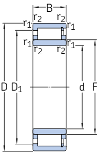
NUH ..ECMH
