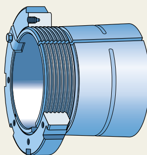
带螺母和防松卡扣的紧定套
