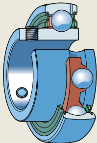
YAT 2 系列轴承
