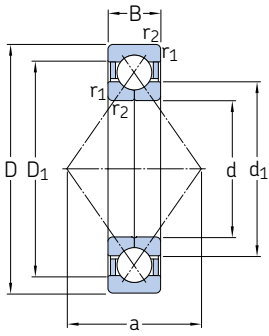
基本系列轴承
