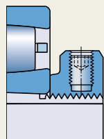
E (带 KMFE 螺母)
