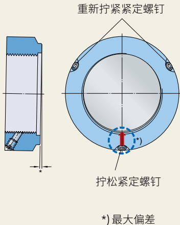
示例 2: KMT 和 KMTA 锁紧螺母调整步骤
