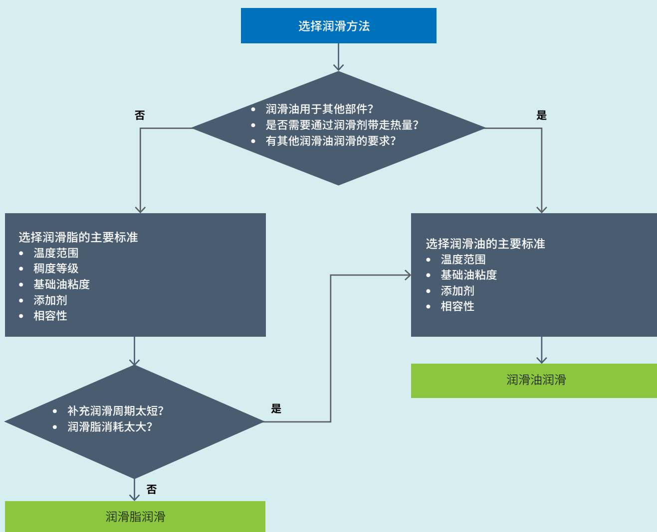
为开式轴承选择合适润滑方法的流程
