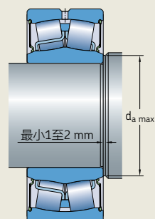
与密封轴承匹配的轴肩
