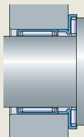
与冲压外圈滚针轴承组合使用的 AXW 系列轴承
