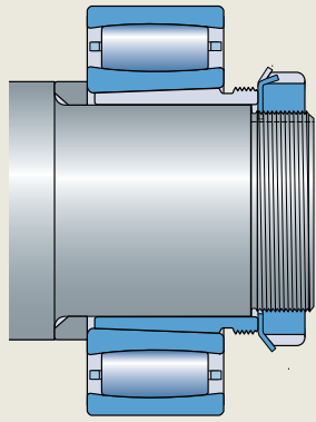
带退卸套的轴承
