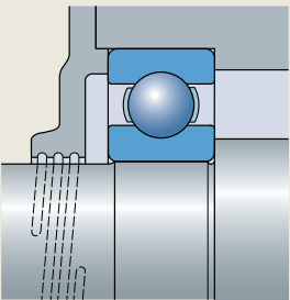
外置带螺旋槽间隙式密封
