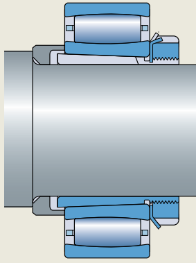
装在阶梯轴上
