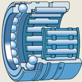
与满装推力球轴承组合，NX
