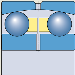
润滑槽和润滑孔
