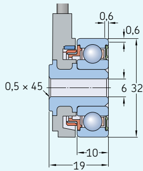
滚轮编码器单元
