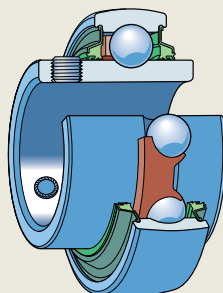
YARAG 2 系列轴承
